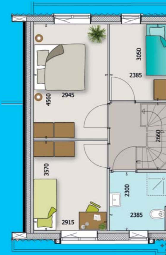
Eerste verdieping
