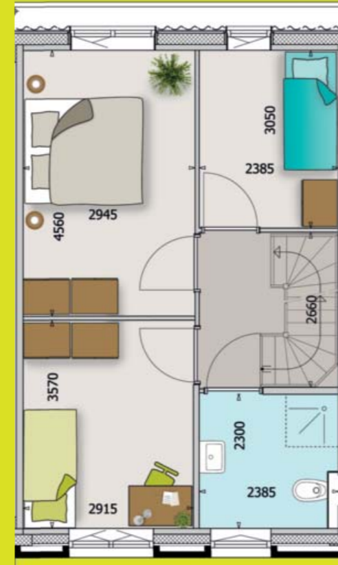
Eerste verdieping
