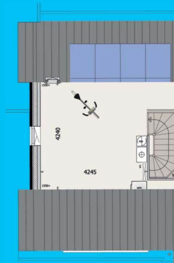
Tweede verdieping
