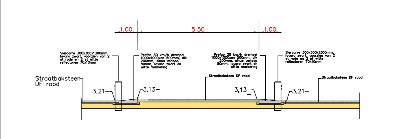
Principe langdoorsnede Prefab verkeersdrempel
