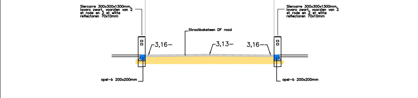
Principe langdoorsnede Prefab verkeersdrempel
